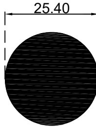
انبوب دائري مصمت قطر 25.4 ملم الرقم التسلسلي للصنف: Y25.4 الوزن 1.378:(Kg/m)
