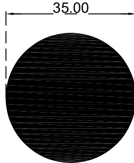
انبوب دائري مصمت قطر 35 ملم الرقم التسلسلي للصنف: Y35 الوزن 2.617:(Kg/m)
