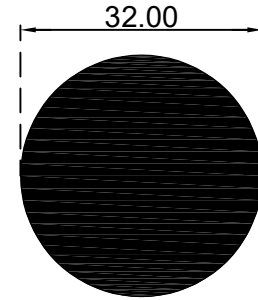
انبوب دائري مصمت قطر 32 ملم الرقم التسلسلي للصنف: Y32 الوزن 2.187:(Kg/m)
