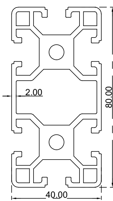
بروفيل طاولة صناعية (40*80) ملم الرقم التسلسلي للصنف: AS00025 الوزن (Kg/m): 2.923
