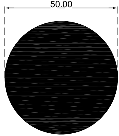
انبوب دائري مصمت قطر 50 ملم الرقم التسلسلي للصنف: YB50 الوزن 5.341:(Kg/m)
