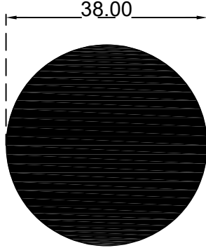
انبوب دائري مصمت قطر 38 ملم الرقم التسلسلي للصنف: Y38 الوزن 3.080:(Kg/m)
