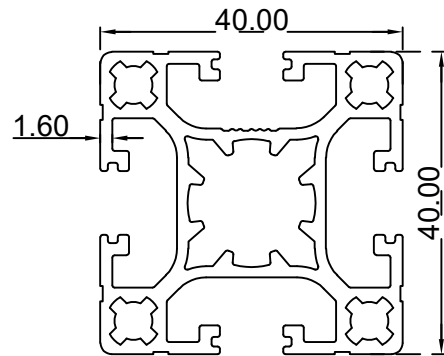
بروفيل طاولة صناعية ثقيل (40*40) ملم الرقم التسلسلي للصنف: BLT3960 الوزن (Kg/m): 1.311
