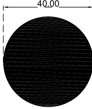
انبوب دائري مصمت قطر 40 ملم الرقم التسلسلي للصنف: Y40 الوزن 3.418:(Kg/m)
