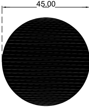
انبوب دائري مصمت قطر 45 ملم الرقم التسلسلي للصنف: YB45 الوزن 4.326:(Kg/m)
