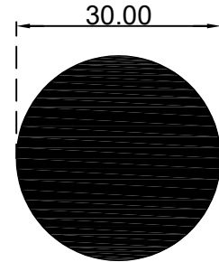
انبوب دائري مصمت قطر 30 ملم الرقم التسلسلي للصنف: Y30 الوزن 1.923:(Kg/m)
